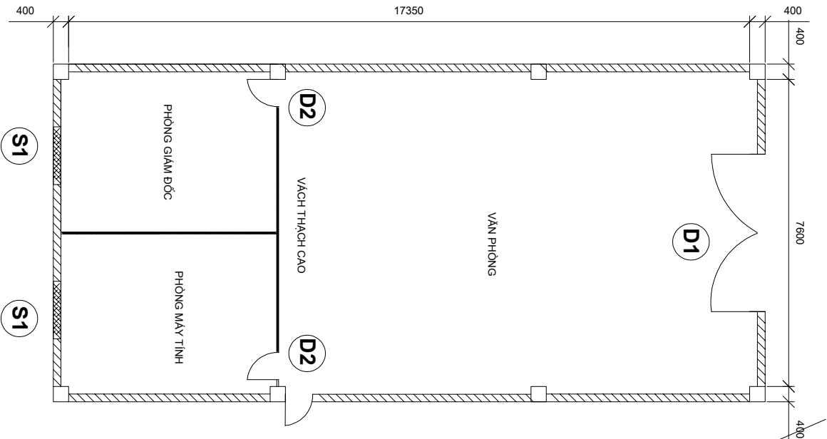
MẶT BẰNG VĂN PHÒNG LÀM VIỆC
